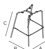
13 gemma - telaio sgabello alto - h.750 ø16 senza tappi gemma - high stool frame - h.750 ø16 without caps
