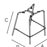
12 gemma - telaio sgabello basso - h.650 ø16 senza tappi gemma - low stool frame - h.650 ø16 without caps
