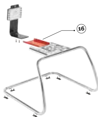
16 piastra adattatore per lama schienale adapter plate for blade back
