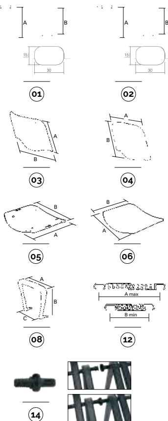
aggancio laterale maschio+femmina in plastica con 2 viti plastic lateral hook male+female with 2 screws 134003-132
