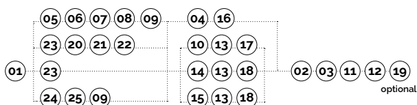
01 square-telaio per sedia fissa senza tappi sottopiede montati square-fixed frame for chair without caps
