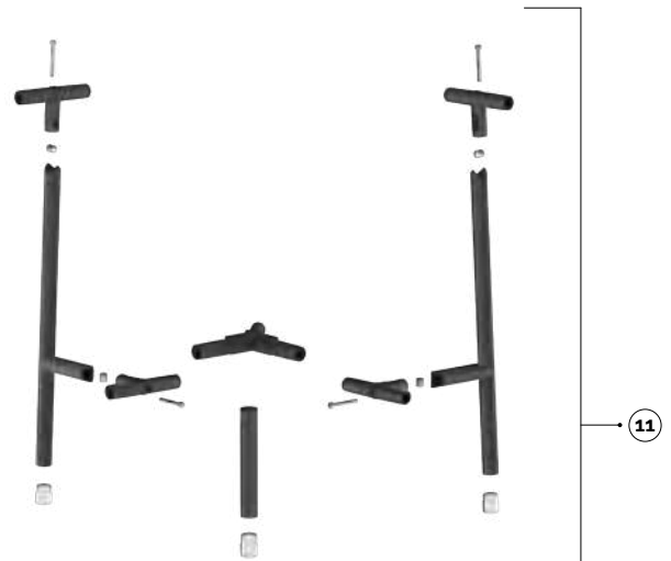
11 unyo.gambe angolari - kit gambe con giunti + piedini + viti unyo.corner legs - leg kit with joints + glides + screws
