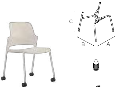
08 genesi - telaio 4 gambe per ruote e piedini alti genesi - fixed 4 legs frame for castors and long glides
