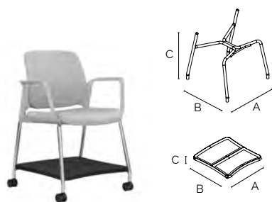
12 genesis - telaio 4 gambe con fori per cestello porta oggetti per ruote e piedini alti genesis - fixed 4 legs frame with holes for storage basket for castors and long glides
