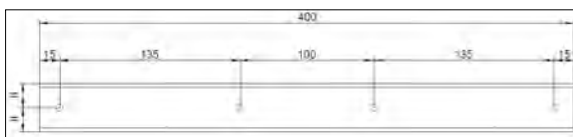
trama di foratura consigliata, lato inferiore trave hole pattern suggested, underneath side of the beam
