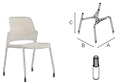
08 genesi - telaio 4 gambe per ruote e piedini alti genesi - fixed 4 legs frame for castors and long glides
