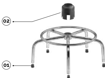
b30-base per sgabello con anello poggiapiedi cono ø50 tappi esclusi b30-base for stool with footrest ring cone ø50 caps excluded
