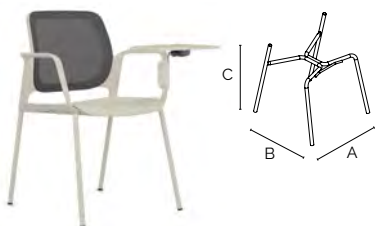
01 genesis - telaio 4 gambe ø.22 senza tappi genesis - 4 legs frame ø.22 without caps
