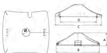
05 cpg-copertina in plastica per telaio girevole cpg-plastic cover for swivel frame
