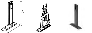
14 90gf-pied fixe pour banquette avec accessoires 90gf-pata fija para banco con accesorios
