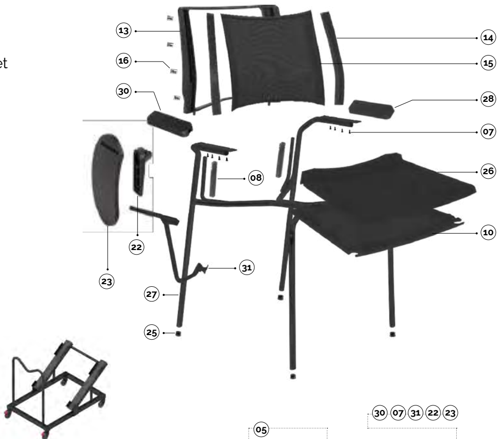
x3-chaîss 4 pieds d.18 avec accoudoirs x3-carro para sillas con accesorios
