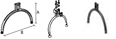
13 100gm-pied mobile pour banquette avec accessoires 100gm-pata móvil para banco con accesorios
