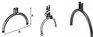
13 100gm-pied mobile pour banquette avec accessoires 100gm-pata móvil para bancada con accesorios
