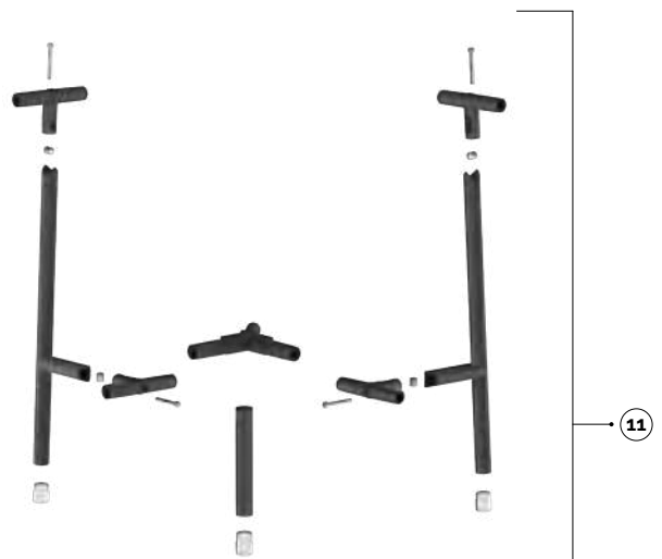
11 unyo.pieds d'angle - kit pieds avec joints + pieds + vis unyo.patas angulaires - kit patas con juntas + pies + tornillos
