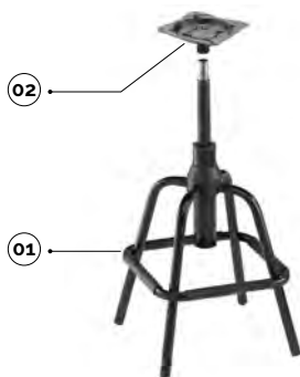
01 sg22-tabourets avec culasse, embouts et accessoires assemblés cône ø21 emballés séparément sg22-taburetes con tornillo grande, tapones y accesorios ensamblados cono ø21 embalaje individual
