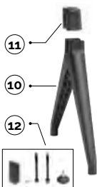
10 jim-pied en plastique noir jim-pata de plástico negra
