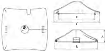
05 cpg-couverture en plastique pour châssis pivotant cpg-cubierta de plástico para estructura versión giratoria
