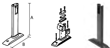
14 90gf-pied fixe pour banquette avec accessoires 90gf-pata fija para bancada con accesorios
