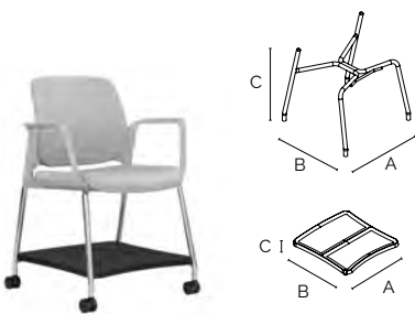
12 genesi - châssis 4 pieds pour roulettes et pieds hauts avec trous pour plateau de stockage genesi - estructura de 4 patas con agujeros para cesto (para ruedas y patas altas)
